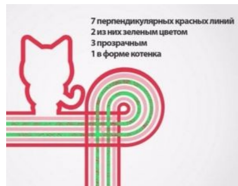
Решение на плоскости
