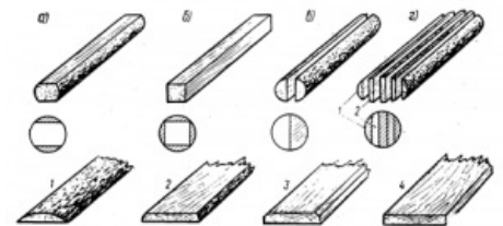
Рис. 6. Пиломатериалы: а — пиленый лес; б — валяк (Прованс, сплюснутый по два канта); в — брусля (Прованс, сплюснутый по четырем кантам); г — планшета (Прованс, распиловка пополам); г — сасса распилы бревна на доски; 1 — горбыль; 2 — необрезан; 3 — полуобрезан; 4 — обрезан
