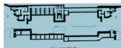
ДОТ Sj-5 «Миллионер» План
