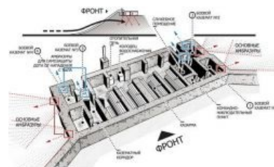
Sn-2 План дота
