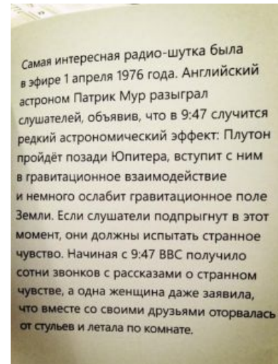
Гравитационное поле Земли
