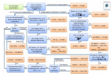
Кодировки.
