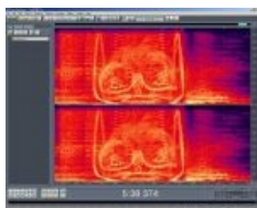
Спираль в «Windowlicker»
